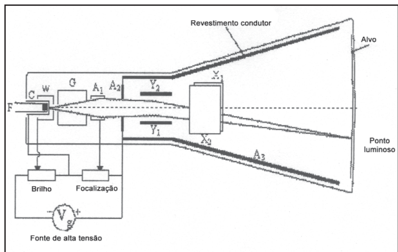
Esquema simplificado de um tubo de raios catódicos, onde F é o filamento de tungstênio, C é o cátodo de um material alcalino, W é a grade de Wehnelt, G, A1 e A2 são ânodos, X1, X2, Y1 e Y2 são os pratos defletores do feixe de elétrons, e A3 é um revestimento condutor. Os pratos defletores direcionam o feixe de elétrons.
